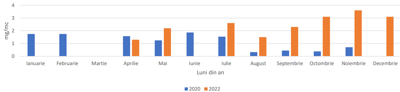
Emisii de H 2 la Cos 7 de captare biogaz, conform rapoartelor de încercare
