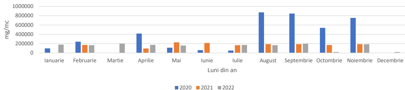
Emisii de CO2 la Cos 1 de captare biogaz, conform rapoartelor de încercare
