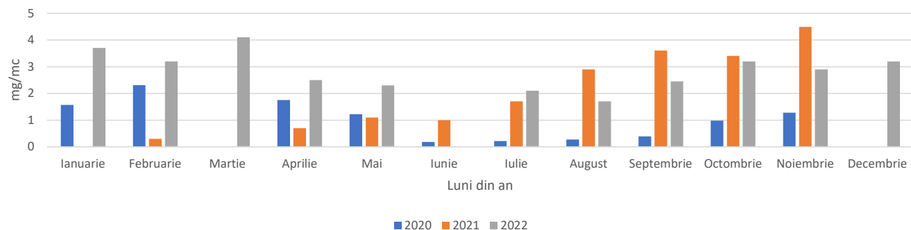
Emisii de H2 la Cos 1 de captare biogaz, conform rapoartelor de încercare
