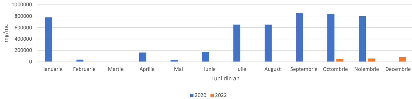
Emisii de CO 2 la Cos 7 de captare biogaz, conform rapoartelor de încercare
