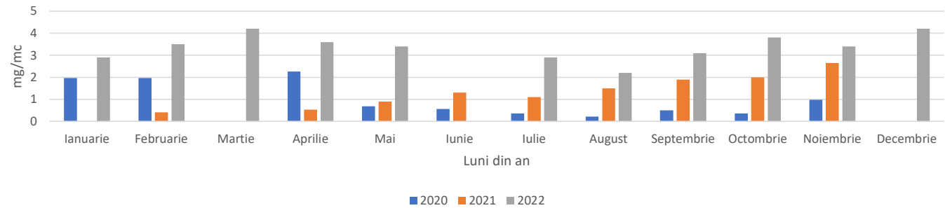
Emisii de H2 la Cos 3 de captare biogaz, conform rapoartelor de încercare
