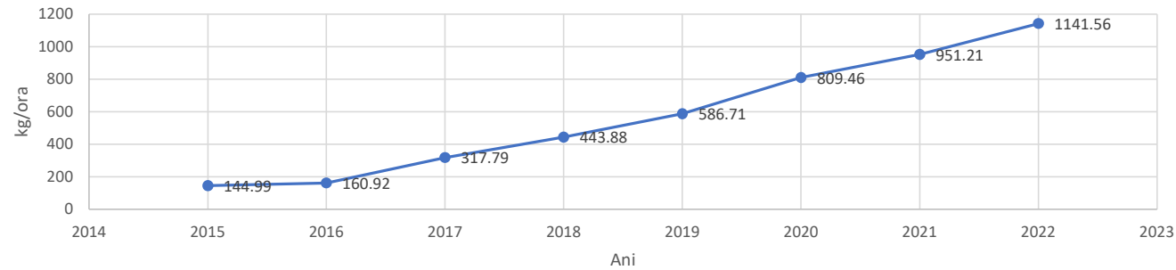
Cantități de emisii dirijate estimate din arderea gazelor la facla - PM10 (kg/ora)
