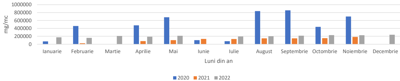
Emisii de CO2 la Cos 3 de captare biogaz, conform rapoartelor de încercare
